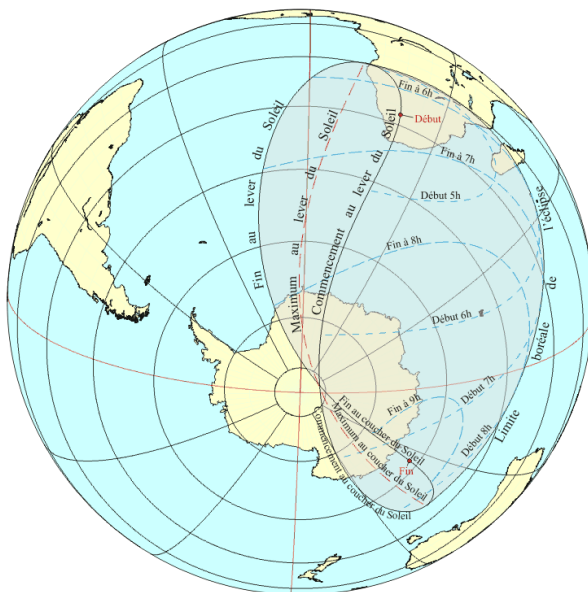
Éclipse partielle du Soleil le 13 septembre 2015
